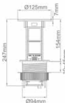
STP-1/4 modules unit
